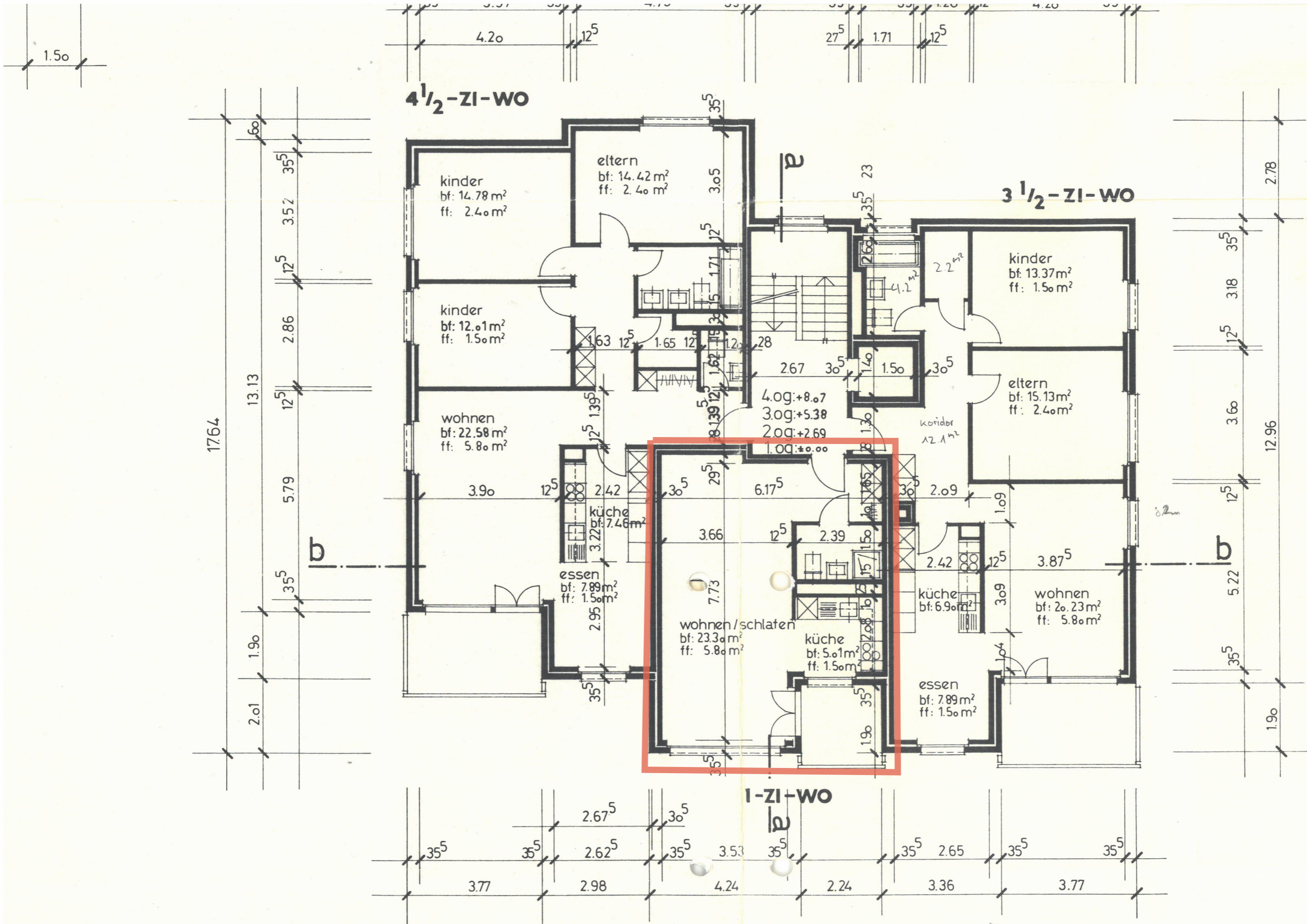
1.- 4. obergeschoss
