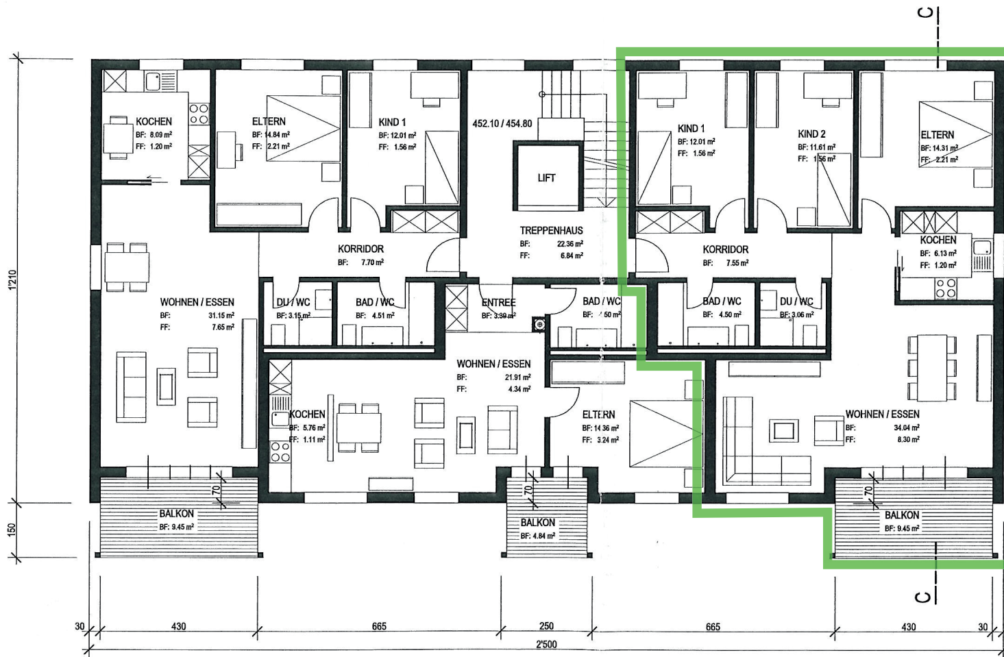
GRUNDRISS 1. / 2. OBERGESCHOSS
